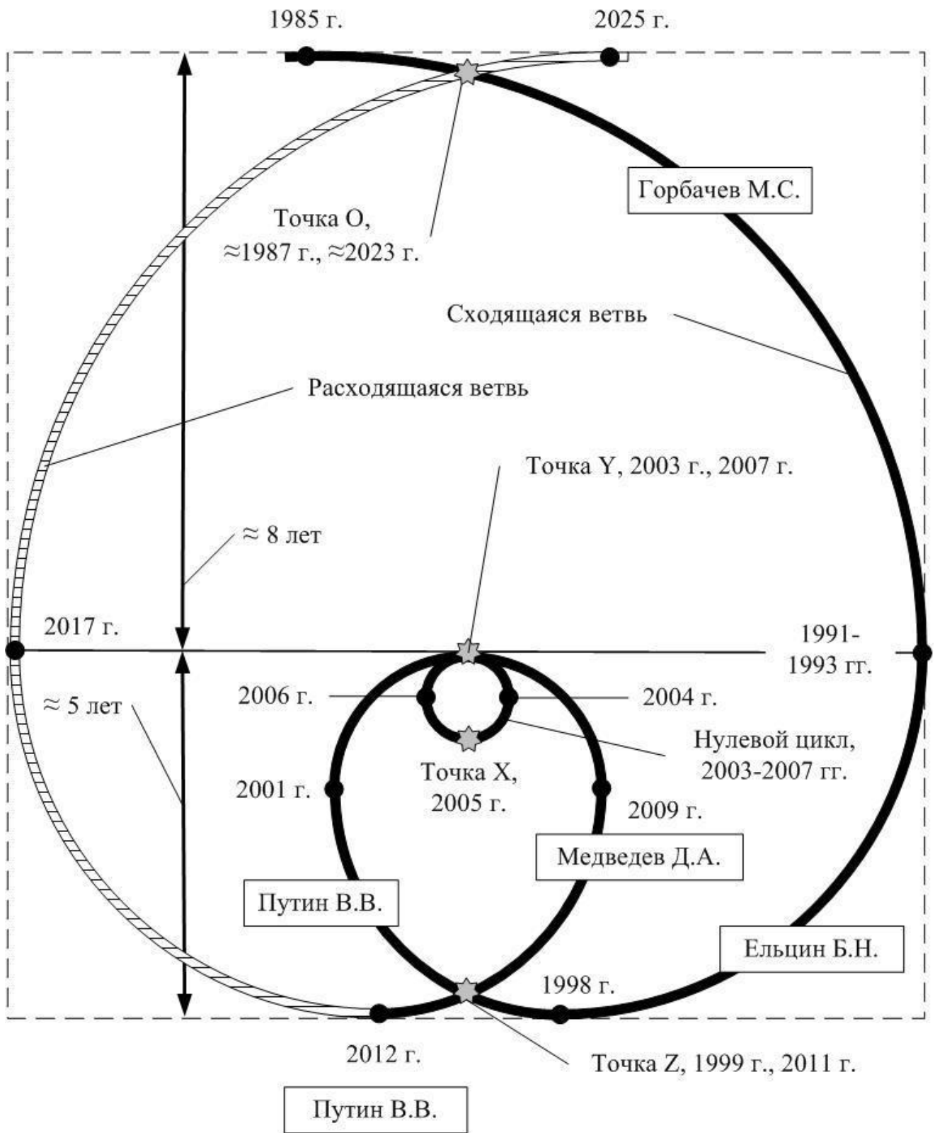
Рис.4. Диаграмма исторических периодов близких к точке X (2005 г.).
