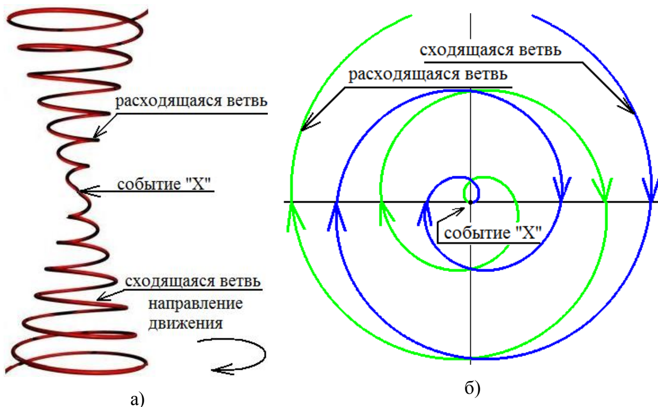
Рис.2. Двойная спираль Фибоначчи с единым фокусом: а) вид сбоку, б) вид сверху.
